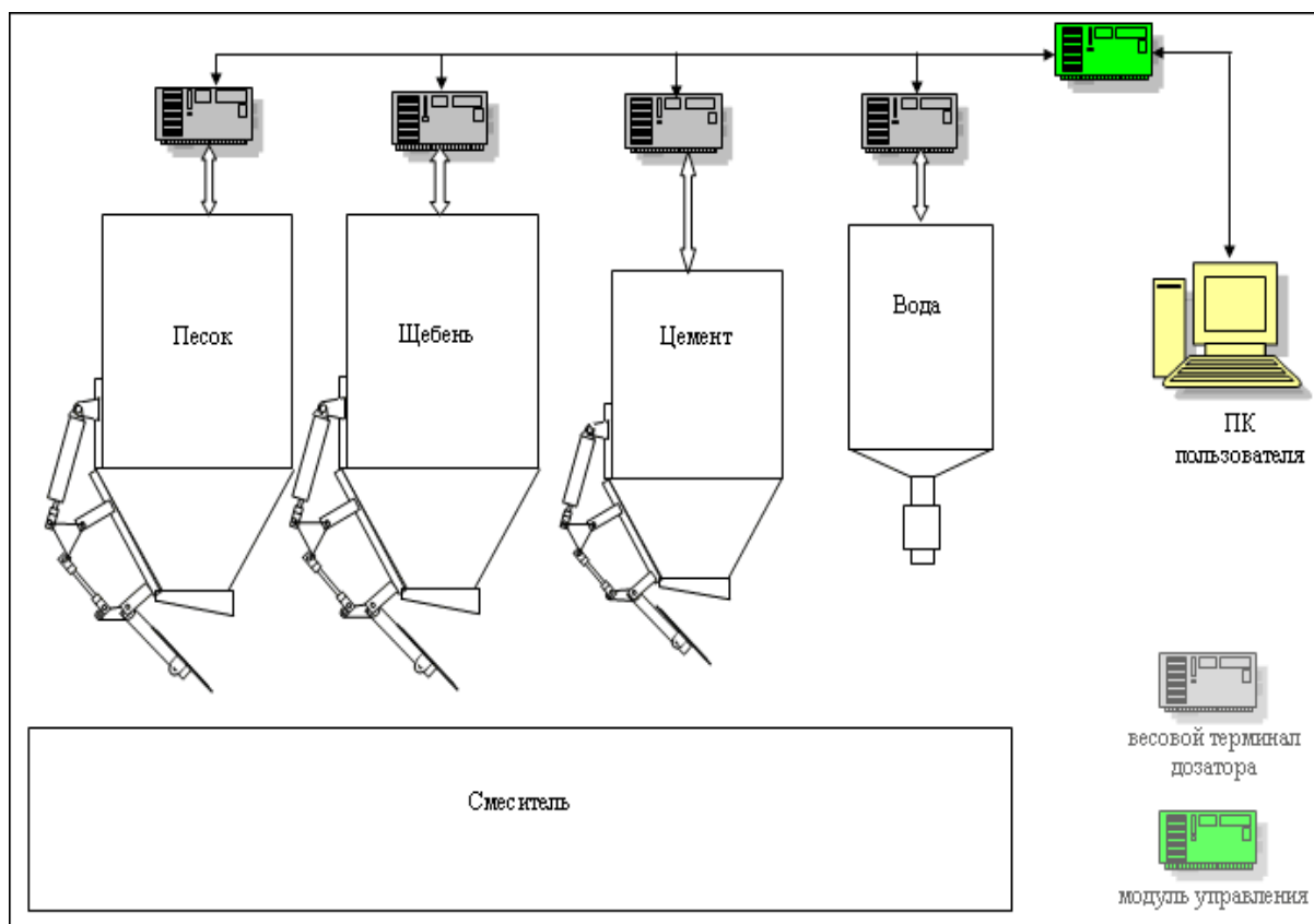
Рисунок 1-Обобщенная схема автоматизации
