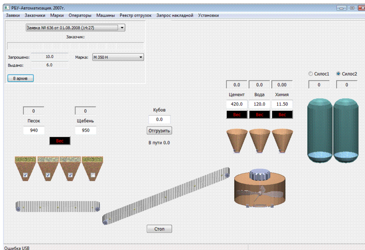
Рисунок 2-Экранная форма системы автоматизации (демо-версия – ярлык «РБУ», пароль доступа - «1»)
